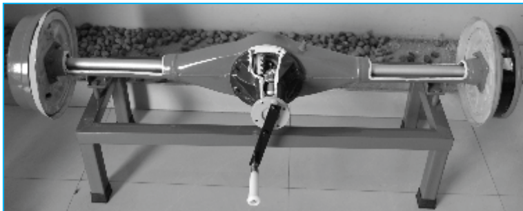
ACTUAL CUT SECTION OF AXLE
